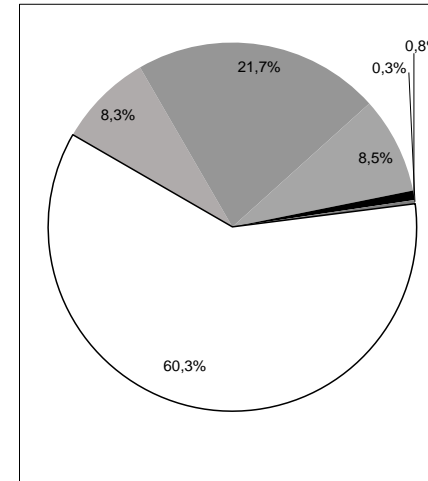
Verbleibender Energieträgermix
